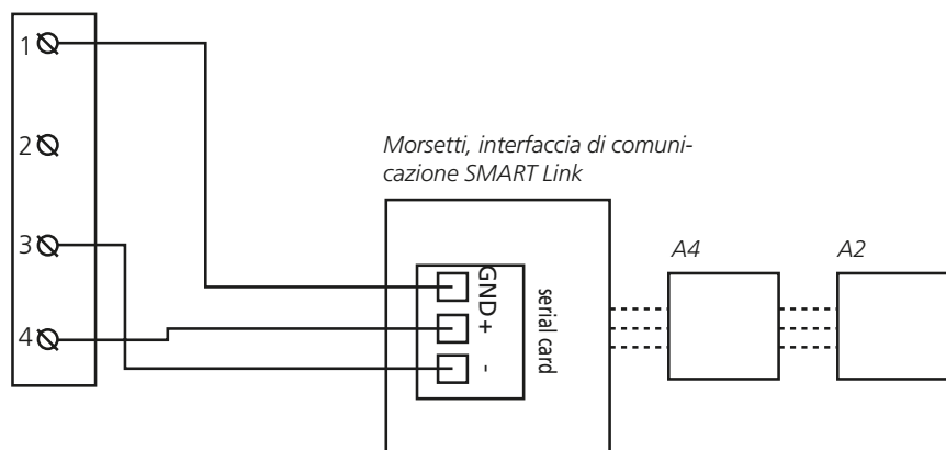
Morsetti per l'adattatore per cavi TBLZ-64
