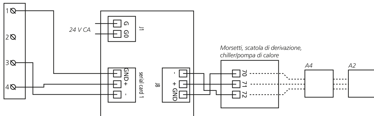
Morsetti, interfaccia di co- municazione SMART Link
