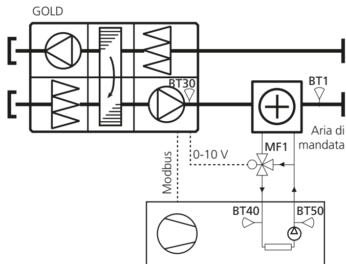
Pompa di calore Swegon È possibile aggiungere una pompa e un serbatoio di accumulo che, a seconda della taglia del sistema, possono essere all'interno o all'esterno della pompa di calore.
