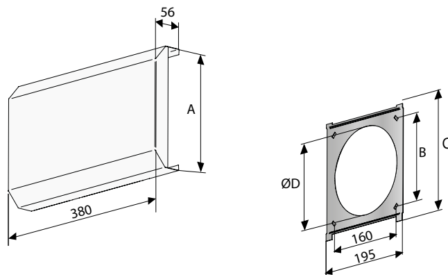
Kuva 4. SOTTO, mitat.
