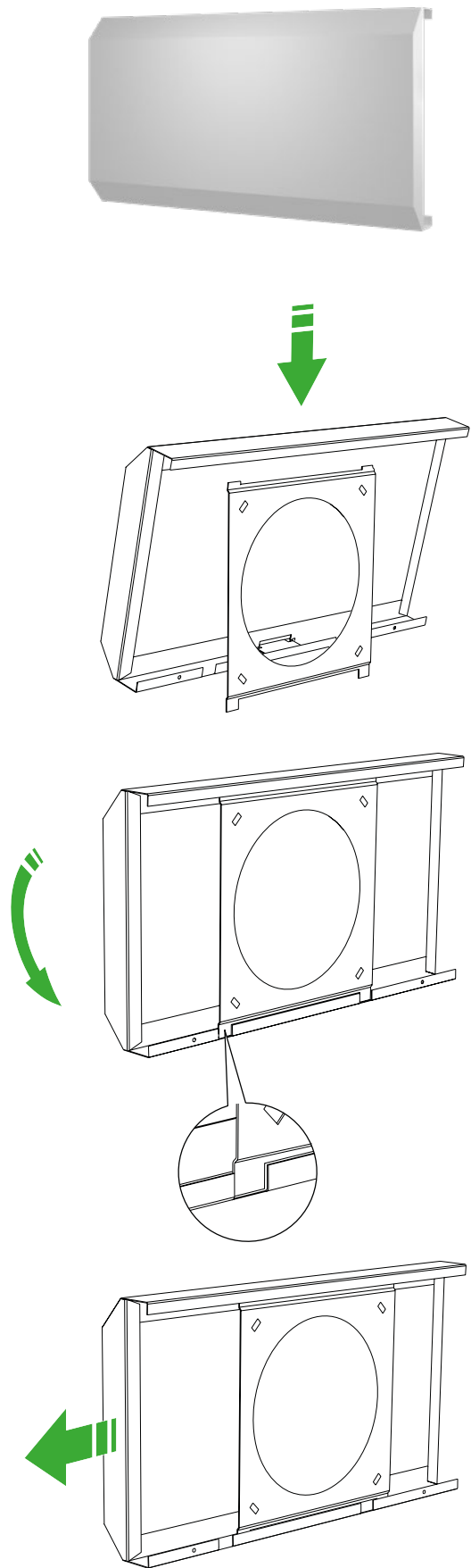
Kuva 1. Asennus.
