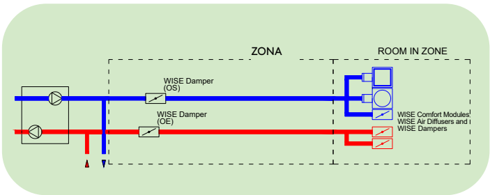
Schema dei circuiti di base, Ottimizzazione della posizione
