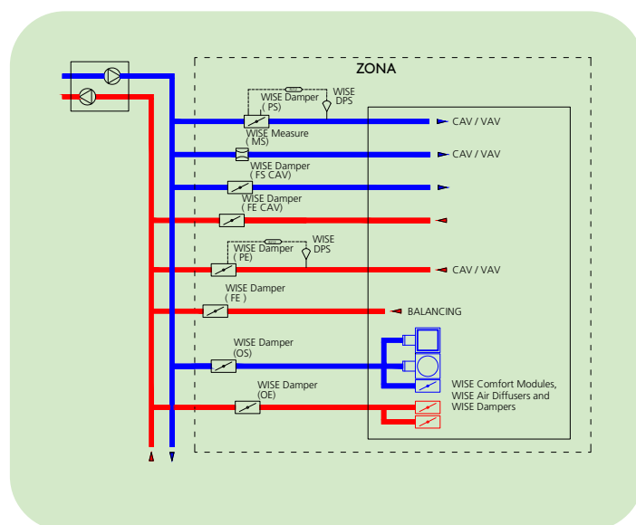
Schema dei circuiti di base, Bilanciamento della portata
