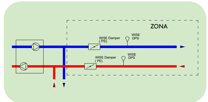
Schema dei circuiti di base, Regolazione della pressione costante
