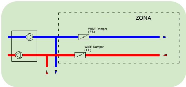
Schema dei circuiti di base, Regolazione della pressione costante
