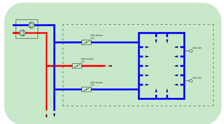
Schema dei circuiti di base, gruppo per la regolazione della pressione costante nei sistemi di canali alimentati ad anello
